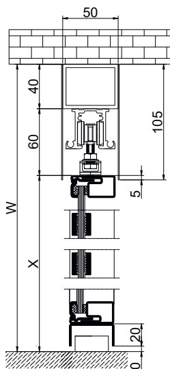
Deckenmontage
