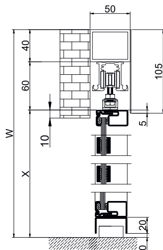
Wandmontage / Sturz
